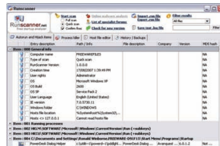
9 RUNSCANNER OPERAČNÍ SYSTÉM WINDOWS 2K/XP/VISTA JAZYK ANGLIČTINA
